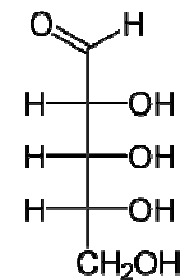
D-Ribose
