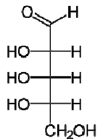
L-Ribose
